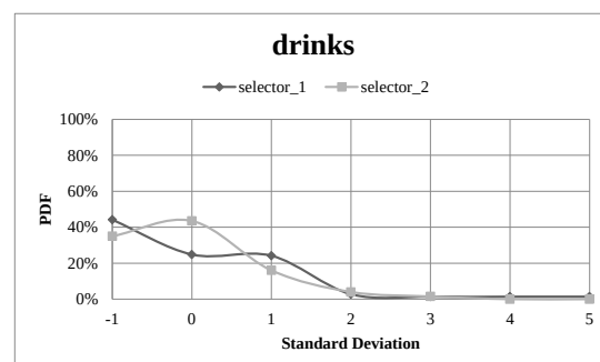
圖 2 Drinks 特徵屬性之機率交集面積
