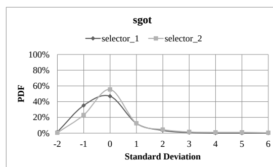
圖 1 GOT 特徵屬性之機率交集面積
