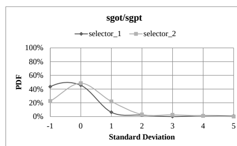
圖 8 GOT/GPT 機率交集面積
