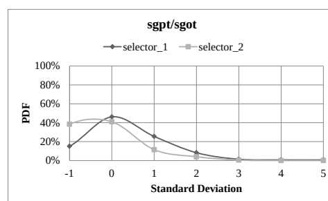
圖 7 GPT/GOT 機率交集面積
