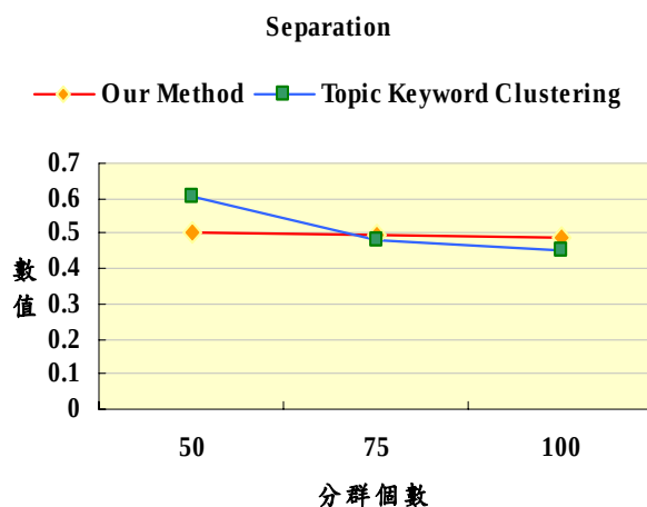
圖 12: Separation 數值之比較
