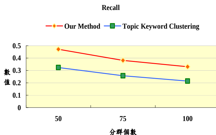
圖 8: Recall 數值之比較
