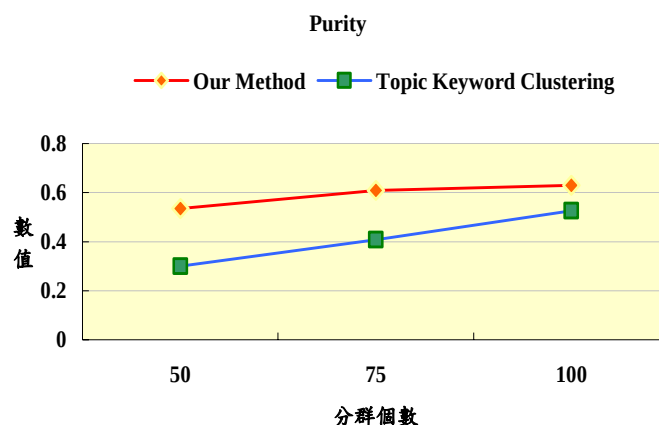
圖 7: Purity 數值之比較
