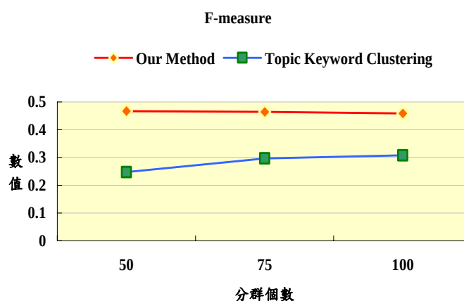
圖 10: F-measure 數值之比較
