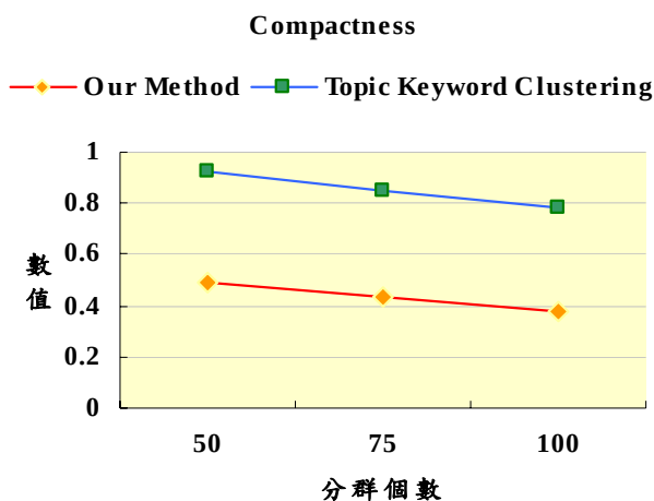
圖 11: Compactness 數值之比較
